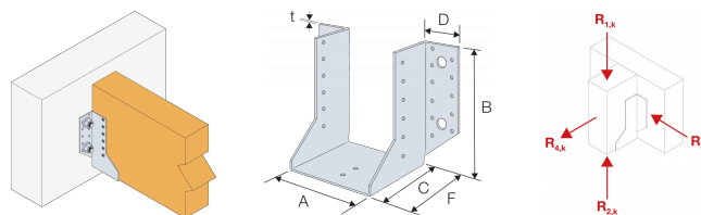
Valeurs Caractéristiques - Bois sur béton ou acier
